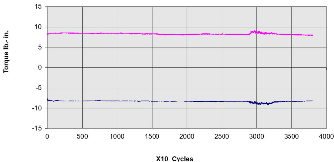
ZE 188 Life Test 38,000 Cycles
